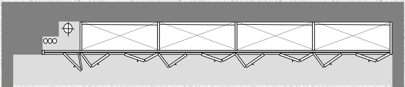
Nischeneinbau von Wand zu Wand
